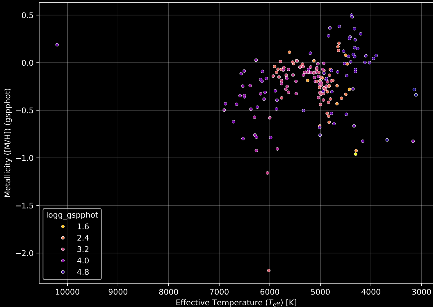
APOGEE DR17 Field: [261+48] Stellar Population Parameters (n= 189)
